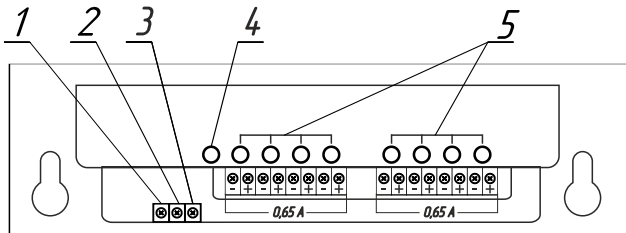
Схема подключения ББП-50 М v8
